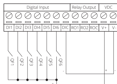
AXM-IO1
