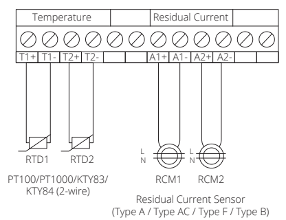
AXM-IO4
